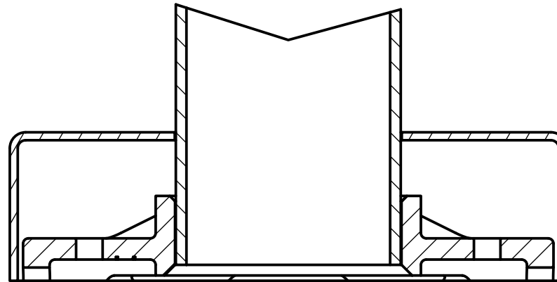
A-A ( 1 : 1 )
