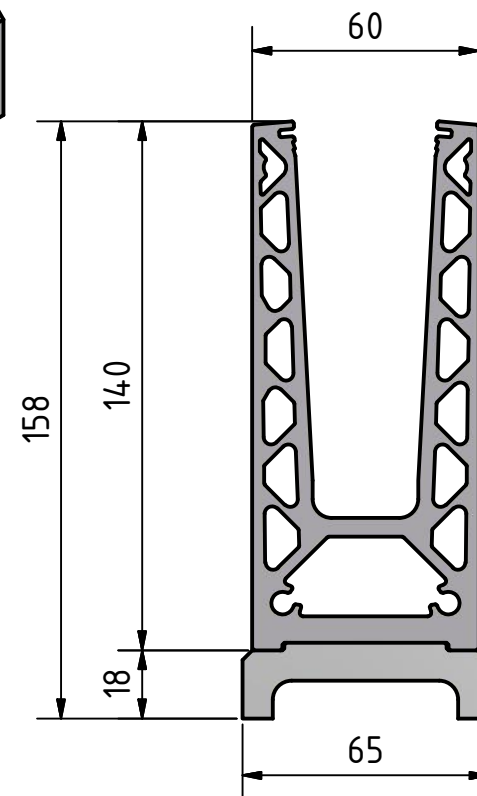
Montage met profiel TL-6020
